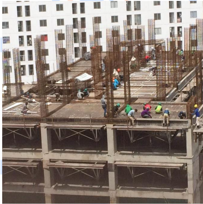
Gambar 3: Pekerjaan di ketinggian, Pemasangan kolom, dan persiapan pengecoran lantai
